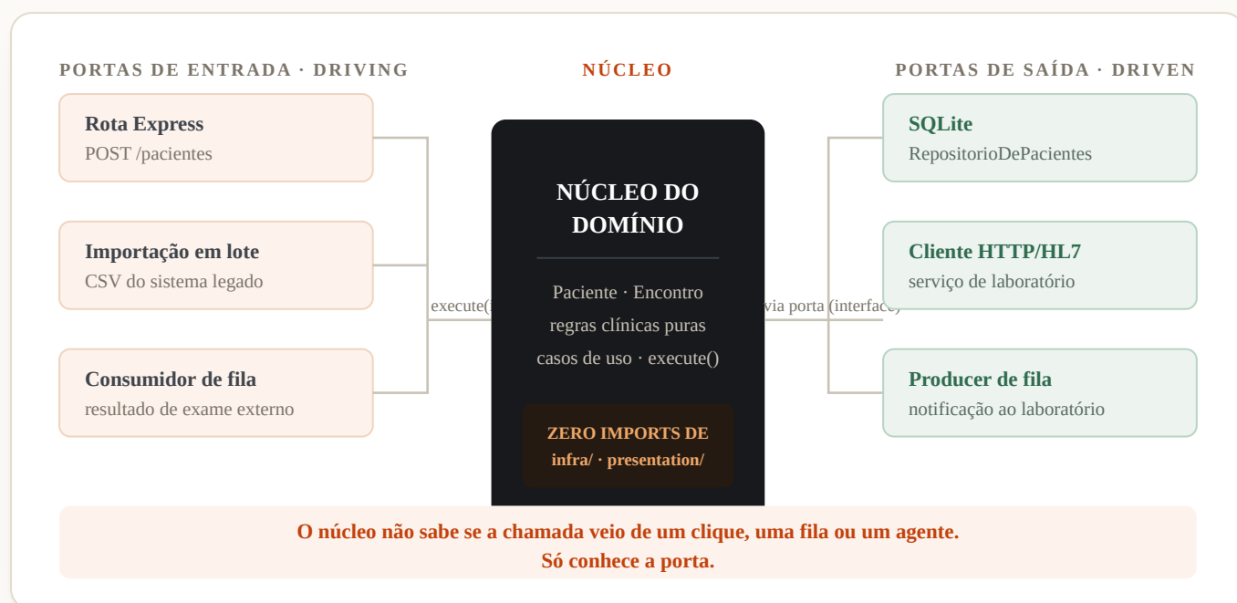
Fig. 1 — Três portas de entrada (driving), três portas de saída (driven), um único núcleo no meio. Cada caixa fora do centro é substituível sem que uma linha do domínio mude — é exatamente essa a promessa que Cockburn fez em 2005 e que continua valendo, agora sob outro nome de urgência.
